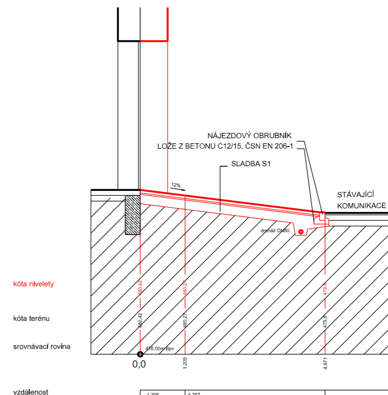
ŘEZ A-A
