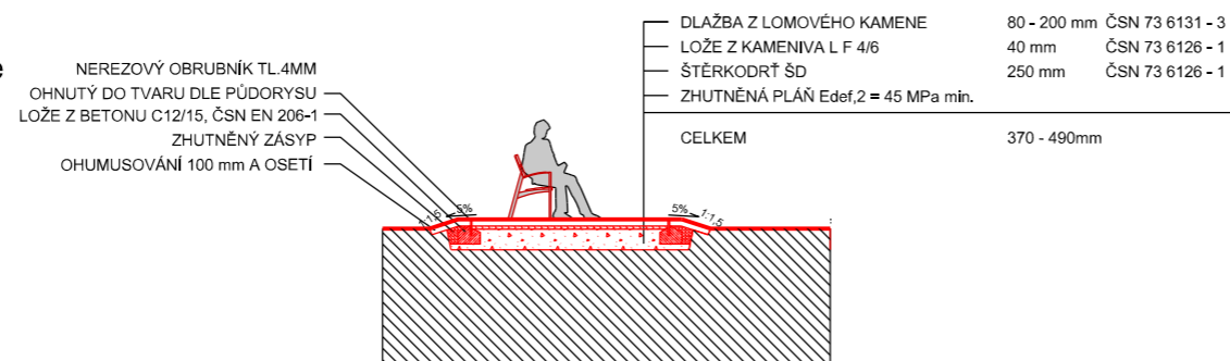
ŘEZ A-A (M 1:100)
