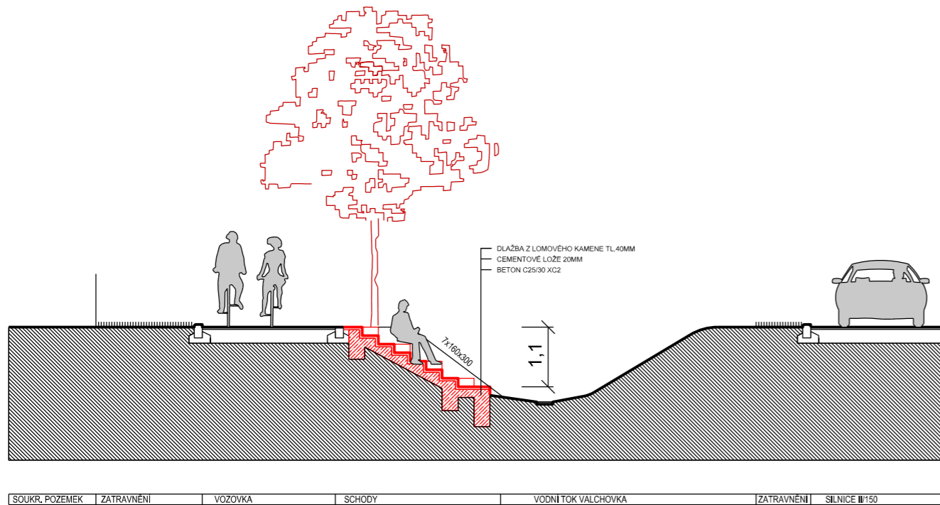
ŘEZ A-A
