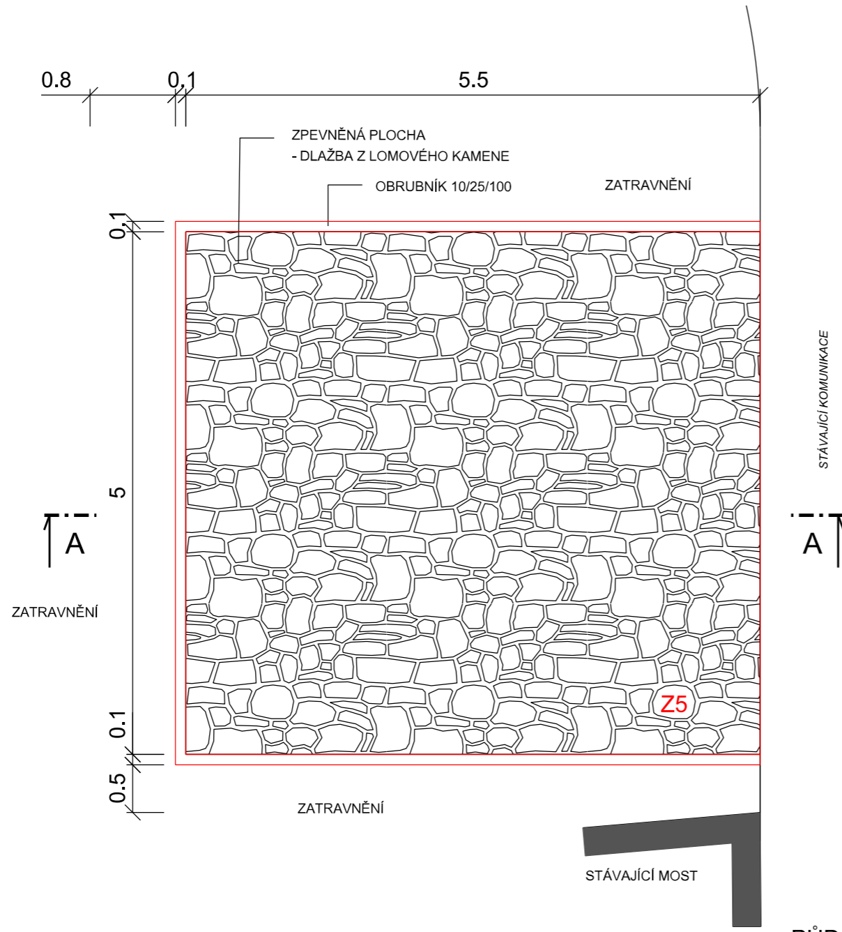
PŮDORYS
