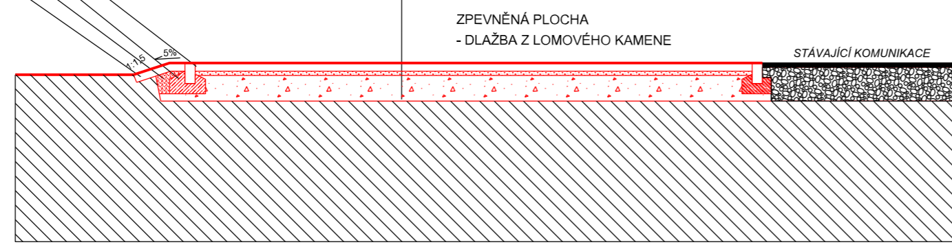
ŘEZ A-A
